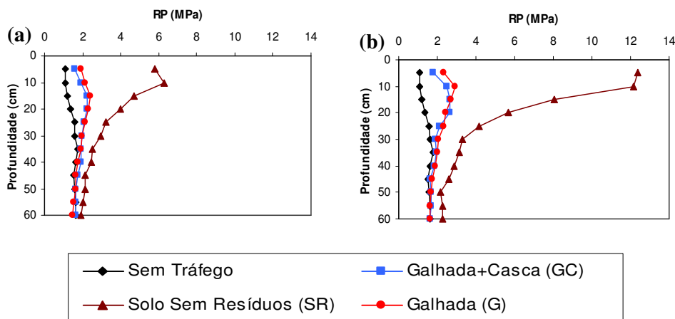
FIGURA 1. Resistência à penetração (RP) em MPa do solo em profundidade em diferentes condições de disposição de resíduos florestais: (a) Região de São João Evangelista, com duas passadas do Forwarder; (b) Região de São João Evangelista, com oito passadas do Forwarder; (Médias de 12 repetições)
