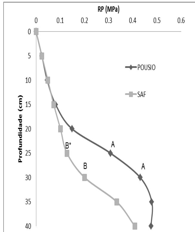
Figura 1- Resistência do Solo à Penetração (RP) em MPa em função da profundidade dos diferentes sistemas de manejo florestal, em Tomé-açu.
