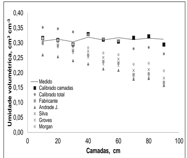
Figura 3. Umidade volumétrica do solo calculada por diferentes equações de calibração de uma sonda de capacitância na camada de 0-100 cm de profundidade de um Latossolo vermelho distrófico.
